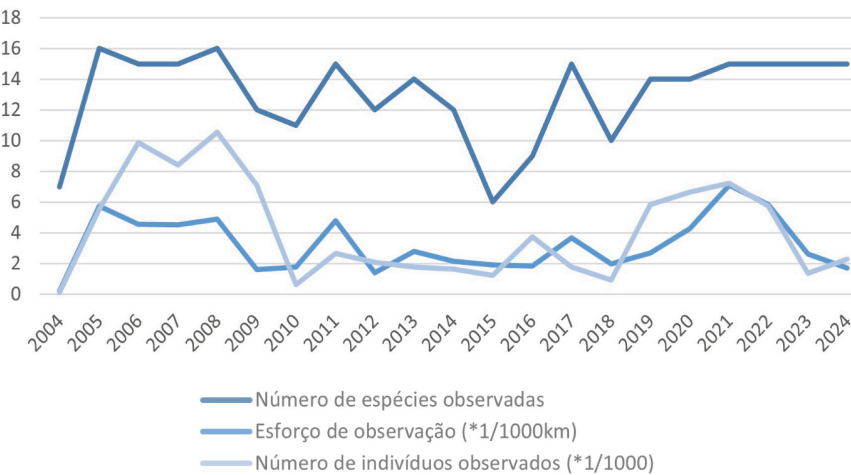
FIGURA 11: Número de km percorridos, espécies-alvo e total de indivíduos observados durante os censos marinhos entre dezembro de 2004 e dezembro de 2024.
